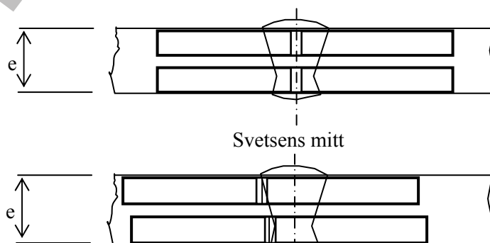
Värmepåverkad zon (HAZ)
